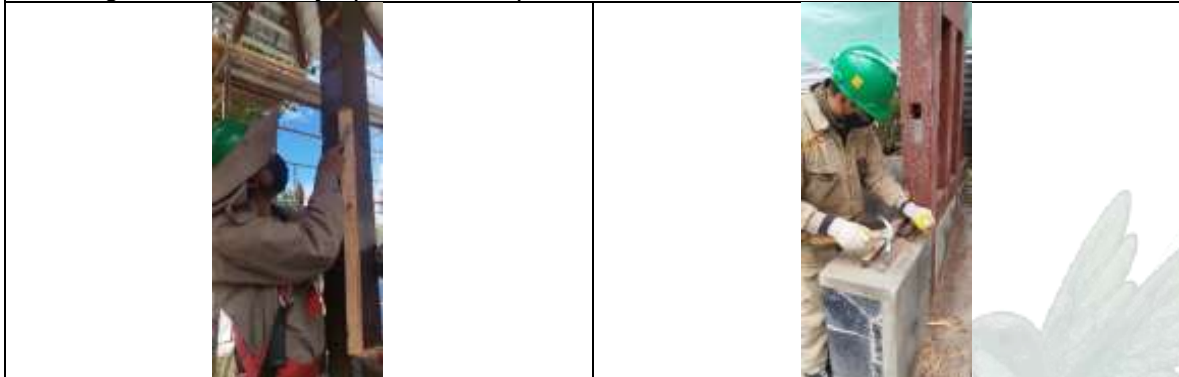
Reintegro de faltantes y aplicación de pintura anticorrosiva de la cubierta de 4 Pórticos
