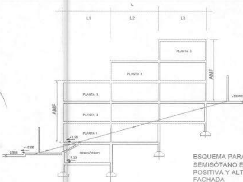
ESQUEMA PARA DEFINICION DE SEMISÓTANO EN PENDIENTE NEGATIVA Y ALTURA MÁXIMA DE FACHADA
