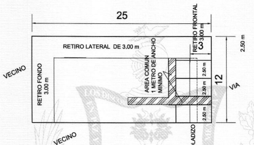
ESQUEMA DE PARQUEOS PRIVADOS SOBRE RETIRO FRONTAL
