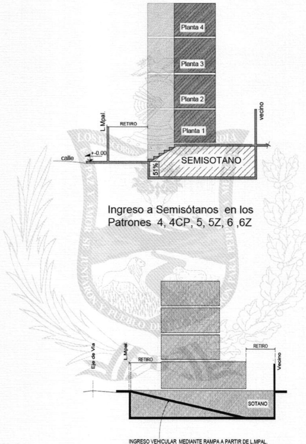
Esquema de Ingreso a Semisótano para Patrones 4, 4CP, 5, 5Z, 6, 6Z.
