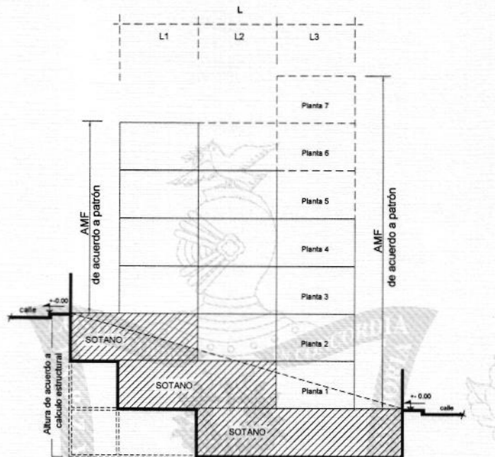
ESQUEMA PARA DEFINICIÓN DE SÓTANO CON DOBLE PATRÓN DE ASENTAMIENTO Y/O DOBLE ACCESO.
