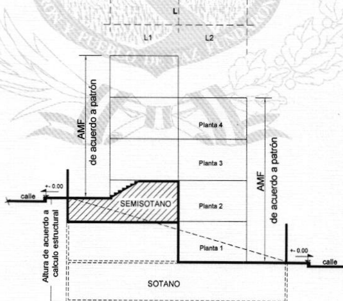
ESQUEMA PARA DEFINICIÓN DE SEMISÓTANO CON DOBLE PATRÓN DE ASENTAMIENTO Y/O DOBLE ACCESO.
